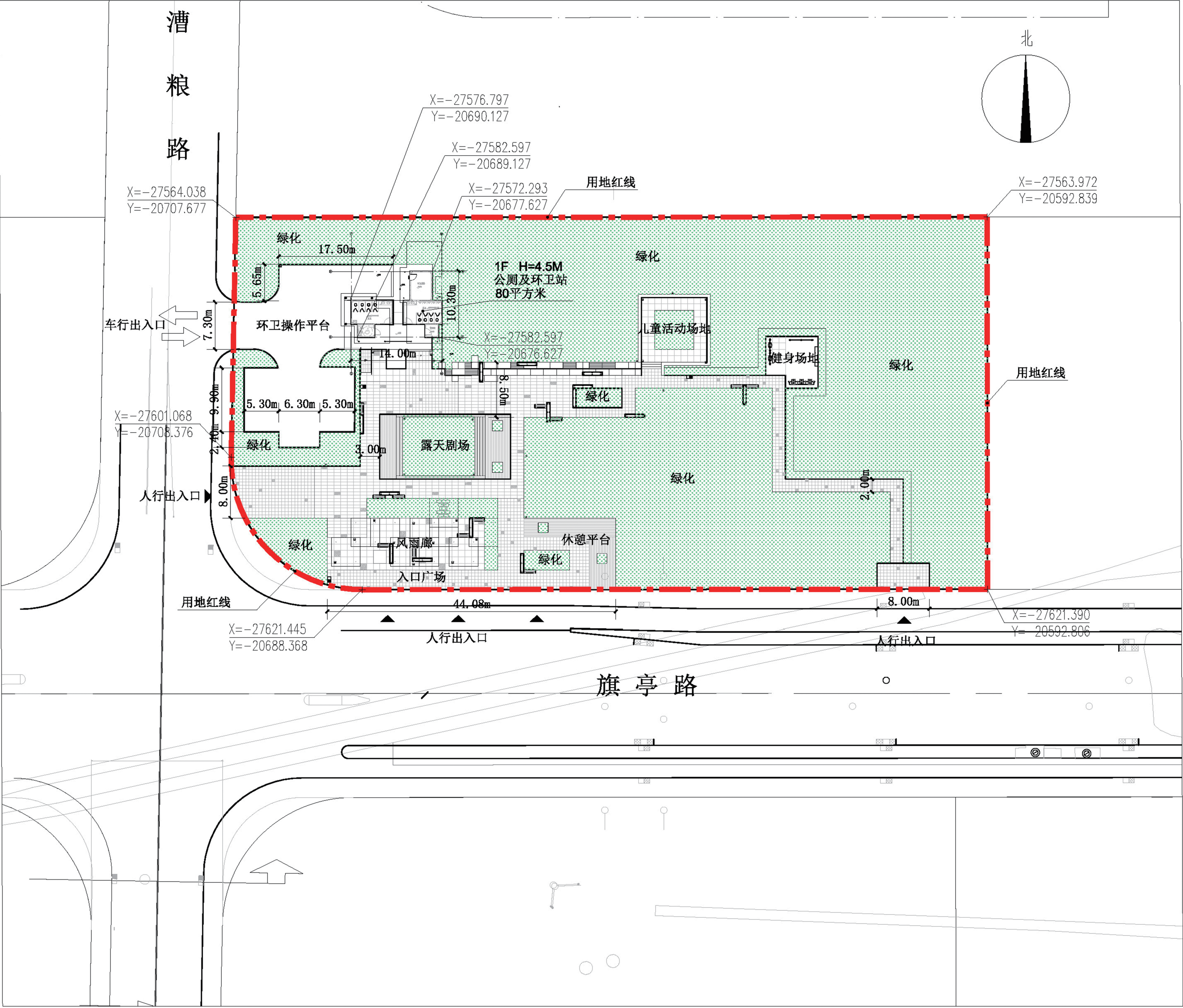
总平面图
